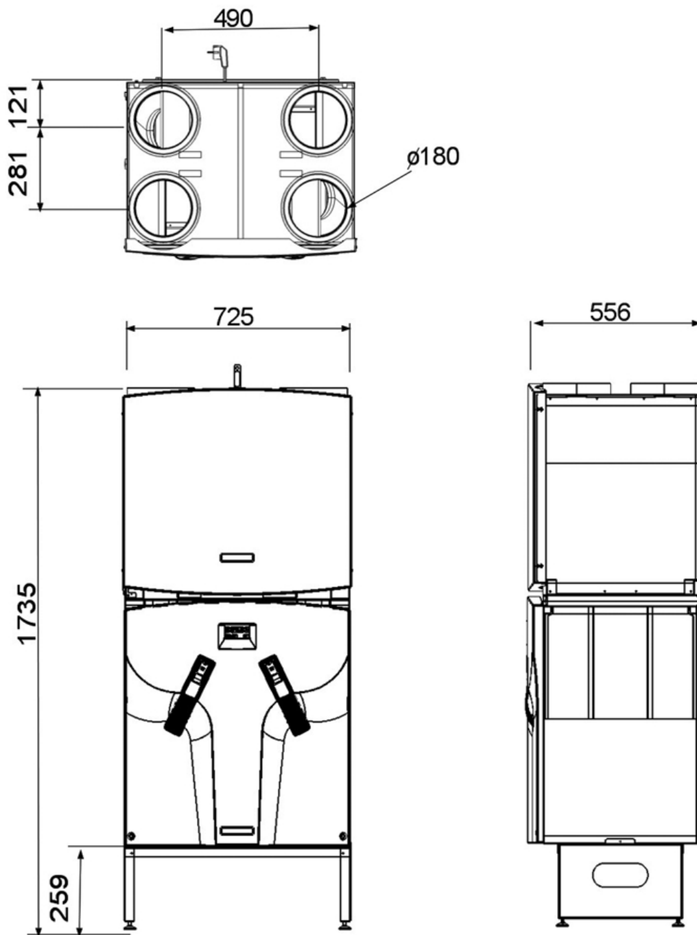
Afbeelding 0.1: ComfoD 550 + ComfoCool 550
